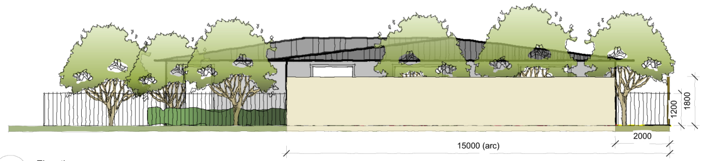
2 Elevation Scale: 1:100
